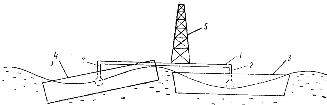
Рис. 1. Тримаран — платформа для бурения на трех качающихся судах-поплавках (вид сбоку). 1 — собственно платформа; 2 — опорные стойки платформы; 3 — кормовые суда-поплавки; 4 — носовое судно-поплавок; 5 — буровая вышка.
