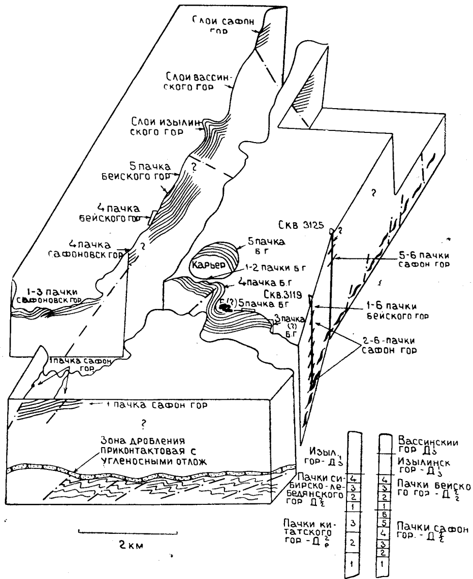
Рис. 2. Блок-диаграмма схематического расположения девонских осадков в надвиговой части Анжерского месторождения (по материалам В. А. Иванни, Е. А. Ивановой, А. З. Юзвицкого)
