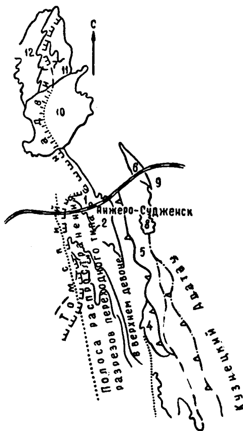
Рис. 1. Схематическая структурная карта северо-восточной части Кузнецкого прогиба. (По материалам Т. Н. Бельской, Н. В. Григорьева, З. А. Мышко, Л. И. Иванчуры, А. З. Юзвического. Цифры означают: 1 — Анжерская синклираль, 2 — Андреевская синклираль, 3 — Низовский синклинорий, 4 — Невский купол, 5 — Яйская глыба (выступ), 6 — Кайтагская синклираль, 7 — Ташминский прогиб, 8 — Золотокитатский грабен, 9 — Яйско-Ишимский выступ, 10 — Улановская впадина, 11 — Новорожденсивенский выступ, 12 — Георгиевское поднятие
