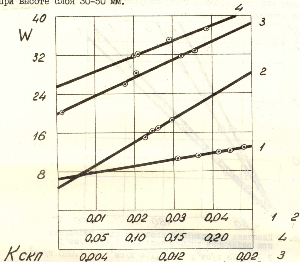
Рис. 2 Зависимости "влагоемкость, % - коэффициент скорости капиллярной пропитки K_{СКП} " для различных материалов.
