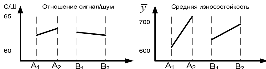
Рис. 5. Воздействие факторов при параметрической оптимизации отношения С/Ш
