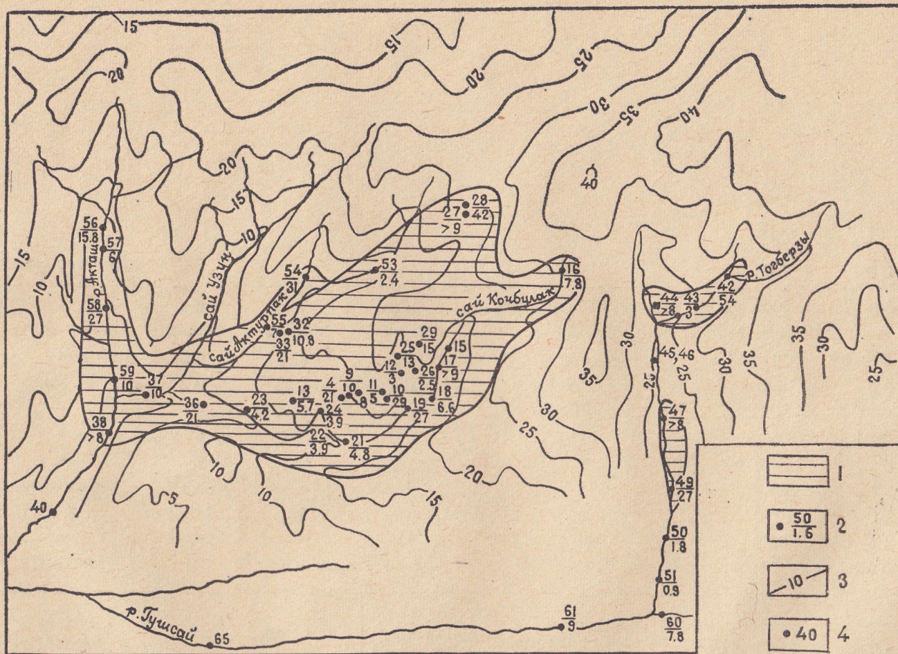
Рис. 1. Поток распространения сурьмы в природных водах золотосульфидных месторождений Кочбулак: 1 — поток распространения подземных вод с содержанием сурьмы более 2 мкг/л; 2 — точка опробования, числитель — номер точки, знаменатель — содержание элемента; 3 — условные горизонталы; 4 — содержание элемента в подземных водах менее 1 мкг/л
