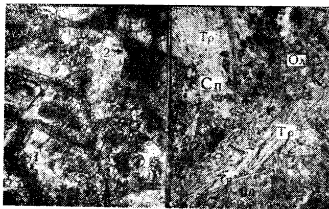
Рис. 4. А — фрагменты микроструктуры оливиновых роговиков
