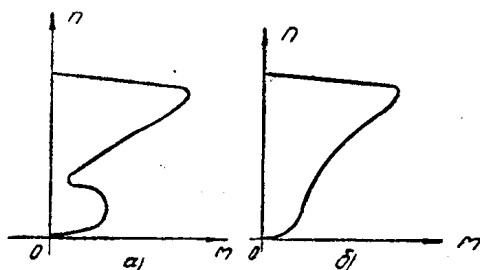
Рис. 2. Опытные механические характеристики ДРС—150 М.
