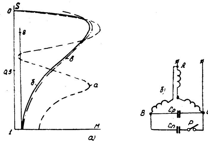
Рис. 1. a — механические характеристики простого, СРД; б — схема соединения конденсаторного ДРС—150М
