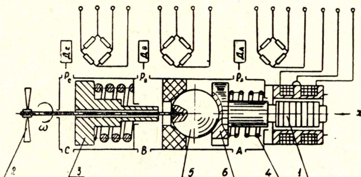
Рис. 1. Принципиальная схема обратного клапана типа ЭКОР и датчиков давлений, перемещения затвора и вращения шарика.
