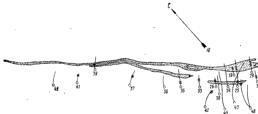
Рис. 1. Выход рудной залежи Бутрахтинского месторождения меди и других металлов на дневную поверхность (закрашен точками) и горизонтальные проекции заложённых для его разведки скважин. Кружками показаны устья скважин. Короткие поперечные прямые соответствуют зонам промышленного оруденения, пройденным скважинами
