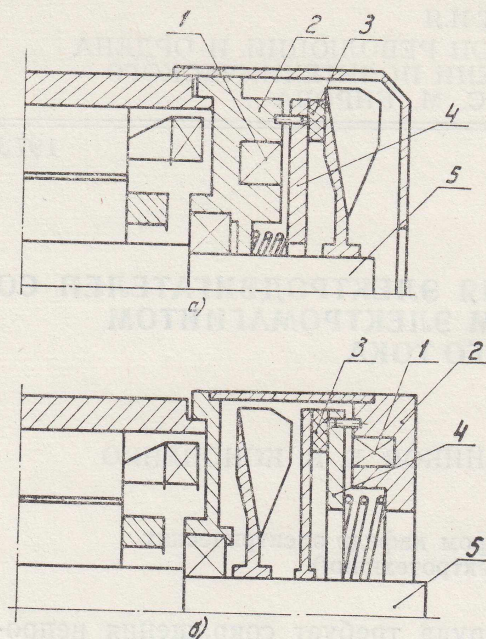
Рис. 1. Схематическое изображение конструкций электродвигателей со встроенным тормозным электромагнитом постоянного тока: а) со встроенным в подшипниковый щит электромагнитом; б) с пристроенным к подшипниковому щиту электромагнитом
