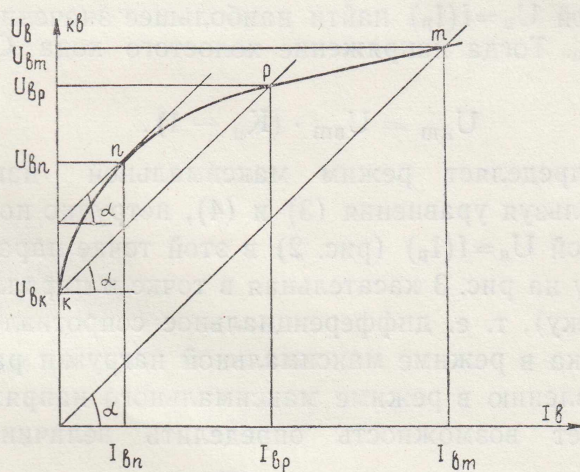
Рис. 2. Вольт-амперная характеристика коронирующего промежутка
