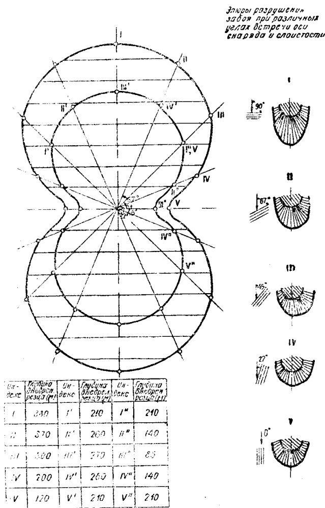
Рис. 2. Диаграмма анизотропии сланцев.
