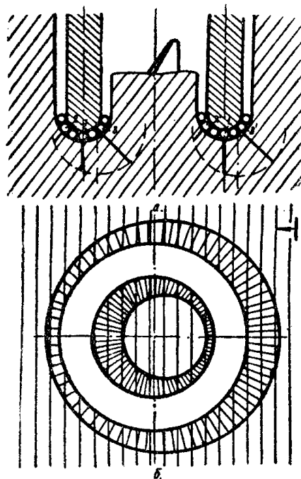
Рис. 1. а) Схема разрушения забоя при колонковом бурении анизотропных пород. б) Эпюра разрушения забоя.
