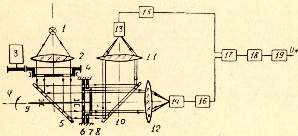
Рис. 1. Схема измерителя параметров углового движения.
