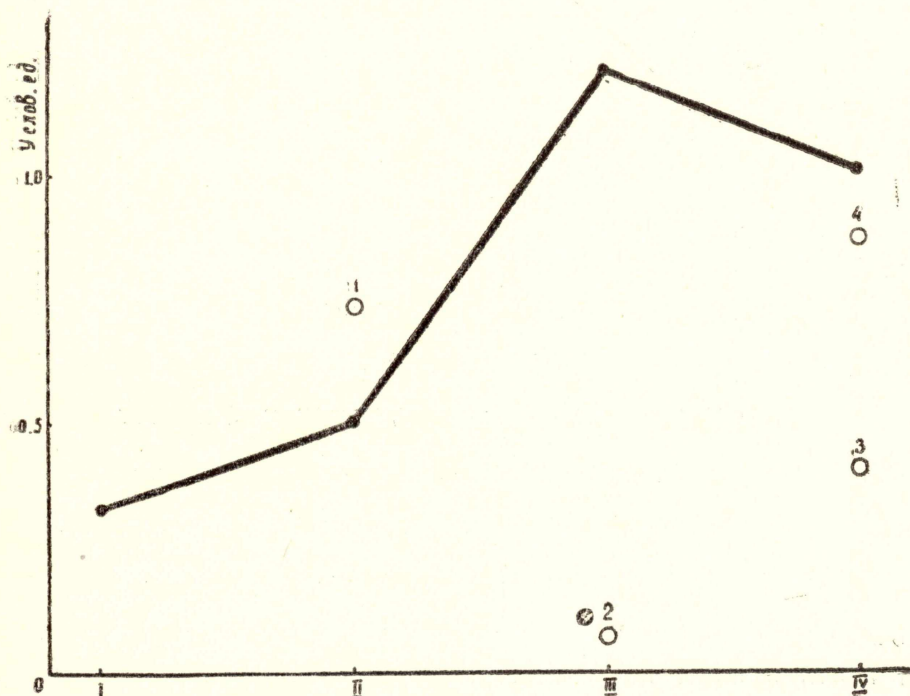
Рис. 1. Радиоактивность акцессорного сфена (в условных единицах) в породах различных интрузивных фаз и в эндоконтактовых образованиях Элекмонарского гранитоидного массива.
