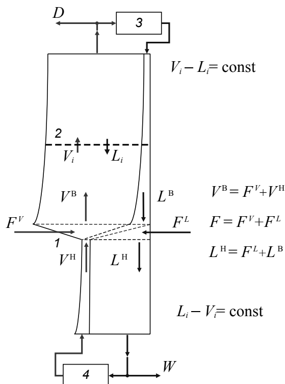
Рис. 1. Схема колонны и потоков жидкости и пара в ней: 1) тарелка питания; 2) контактное устройство; 3) дефлегматор; 4) кипятильник. Расходы: F , F^V , F^L – питания полный, в паровой и жидкой фазах, соответственно; V_i , V^B , V^H – пара в i -ом сечении колонны, в верхней и нижней частях колонны, соответственно; L_i , L^B , L^H – жидкости в i -ом сечении колонны, в верхней и нижней частях колонны, соответственно; D – дистиллята; W – кубового остатка
