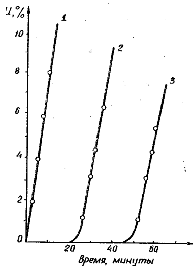
Рис. 3. Кинетика полимеризации 3-метил-9-ВК в присутствии бензохинона при 75°: 1 — без ингибитора; 2 — конц. бензохинона 1,47 \cdot 10^{-3} моль/л; 3 — конц. бензохинона 2,95 \cdot 10^{-3} моль/л.
