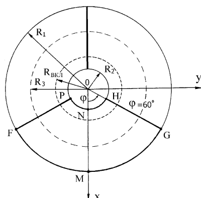
Рис. 2. Геометрические параметры секторов ведущего устройства. FPNHGM – один из трёх секторов; MNHG – рассчитываемая половина сектора
