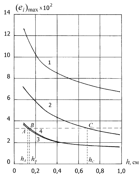
Рис. 4. Зависимости максимальных значений интенсивности деформаций (e_i)_{\max} в секторе ВУ от геометрических параметров вкладышей
