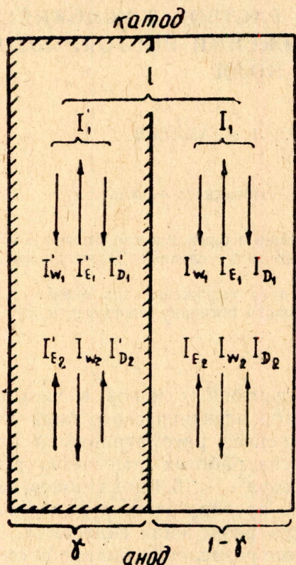
Рис. 1. Схема потоков при разделении ионов противоточной электромиграцией в системе ионит — раствор: [////] — фаза ионита, [ ] — фаза раствора.
