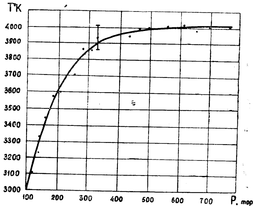
Рис. 2. Зависимость газовой температуры плазмы смеси воздуха с продуктами разложения полимеров от давления.
