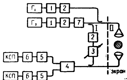
Рис. 3. Блок-схема установки для микроволновых исследований.
