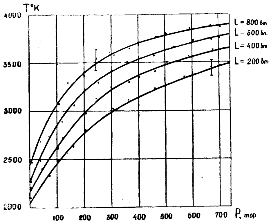
Рис. 1. Зависимость газовой температуры факельного разряда в воздухе от давления при различных мощностях, вкладываемых в разряд ( L=200, 400, 600, 800 вт).
