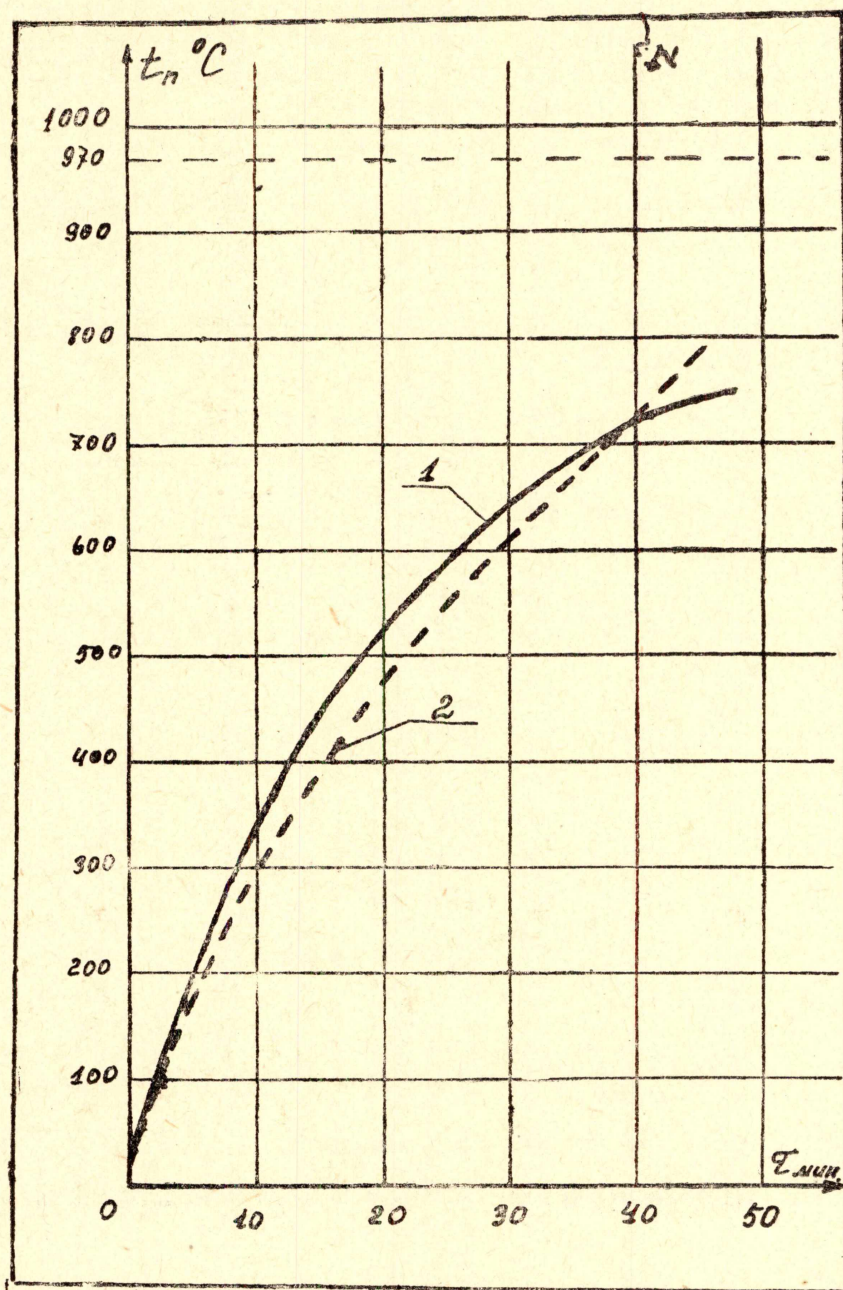
Фиг. 1. Прогрев цилиндра из стали 9X диаметром 300 мм: 1. Изменение температуры на поверхности по данным опыта [2]. 2. Изменение температуры на поверхности при тех же условиях, построенное по формуле (8).
