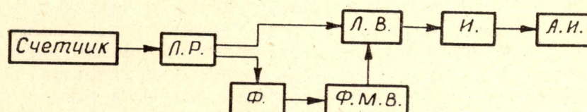
Рис. 1. Блок-схема установки уровней дискриминации формирователей.
