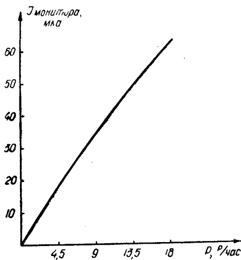
Рис. 5. Зависимость показаний монитора от величины мощности дозы тормозного излучения
