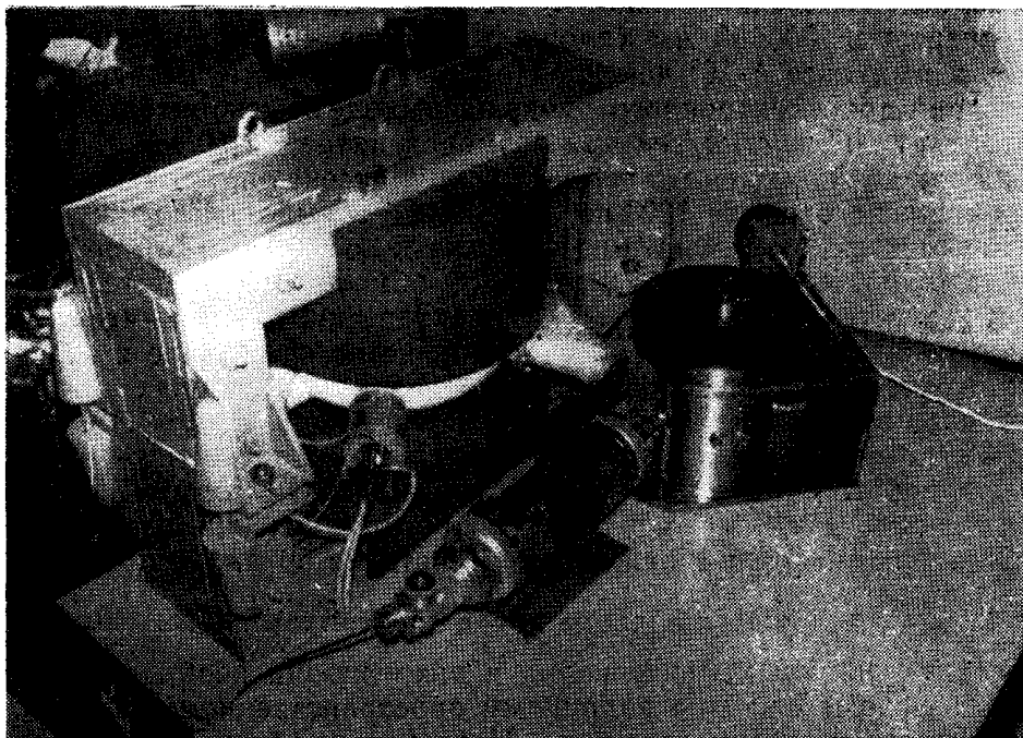
Рис. 1. Внешний вид бетатрона на 6 Мэв с выводом электронного пучка
