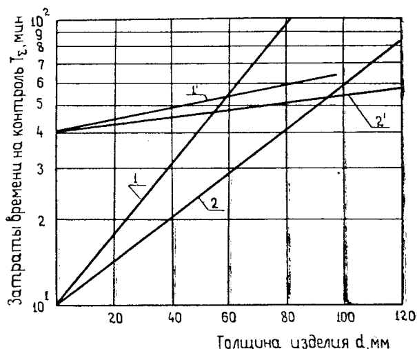
Рис. 1. Зависимость затрат времени от толщины поглотителя (1, 1' — алюминий, 2, 2' — магний) при рентгенографировании на термолюминесцентный преобразователь (1, 2) и рентгеновскую пленку РТ-1 (1', 2')
