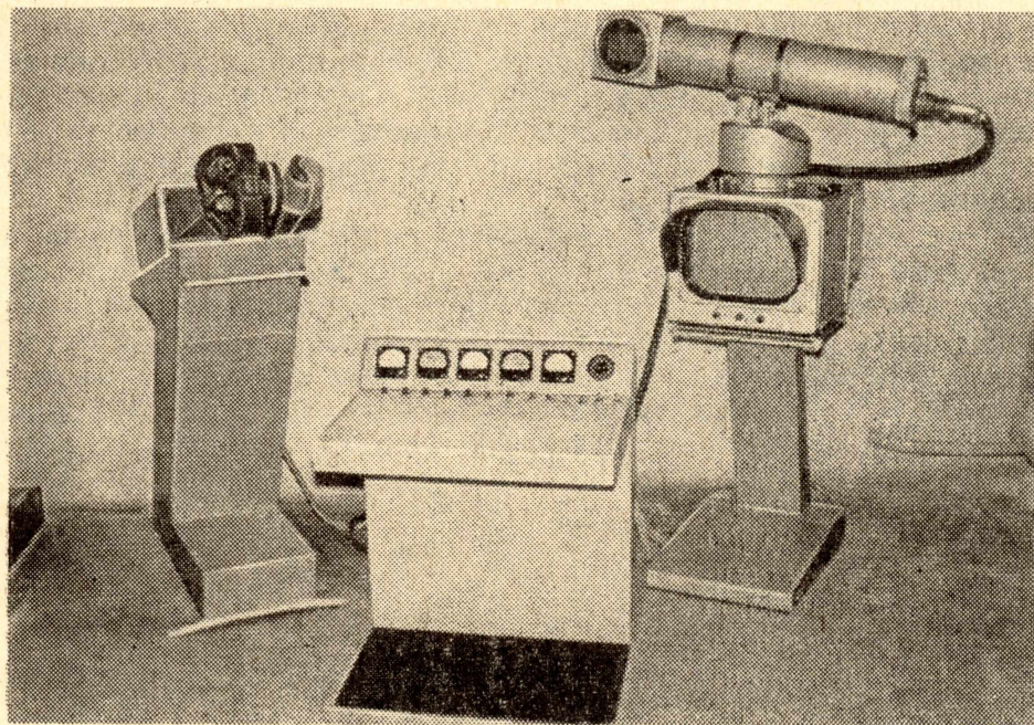
Рис. 4. Интроскоп для наблюдения и кинорегистрации динамических процессов
