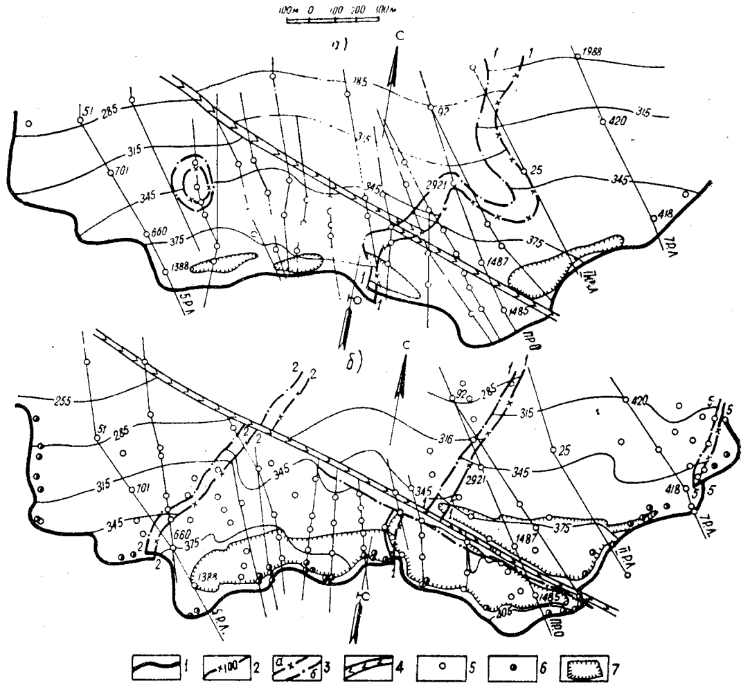
Рис. 2. Структурная карта пласта .IV—V по данным геологоразведочных (а) работ (1961) и по данным геологоразведочных и эксплуатационных (б) работ (по состоянию на 1966 г). Условные обозначения: 1 — выход угольного пласта угля; 2 — изогипсы почвы пласта угля; 3 — обрывы пластов тектоническими разрывами: а — лежащего крыла, б — висячего крыла; 4 — дайка диабазов; 5 — скважины колонкового бурения; 6 — дудки; 7 — отработанные участки пласта
