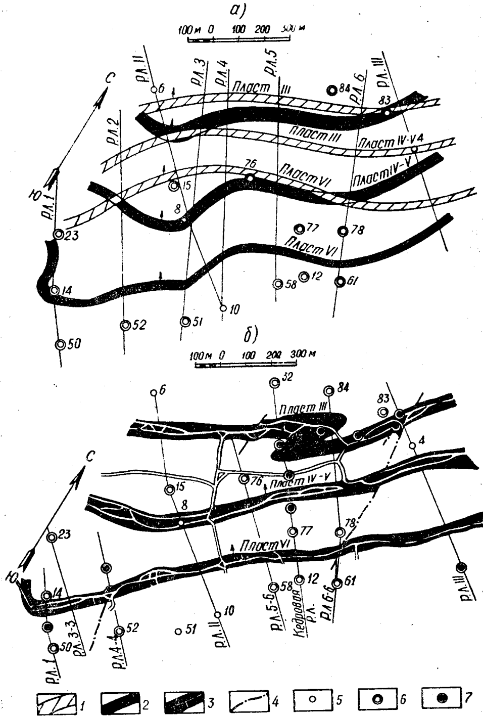
Рис. 1. Пластовая карта гор.+245 м по данным: а) предварительной (1946 г.) и детальной (1949 г.) разведок; б) доразведки и эксплуатации. Условные обозначения: увязка угольных пластов по данным: 1 — предварительной разведки; 2 — детальной разведки; 3 — доразведки и эксплуатации; 4 — дизъюнктивы; 5—7—скважины колонкового бурения, пробуренные: 5 — на стадии предварительной разведки, 6 — на стадии детальной разведки; 7 — при доразведке
