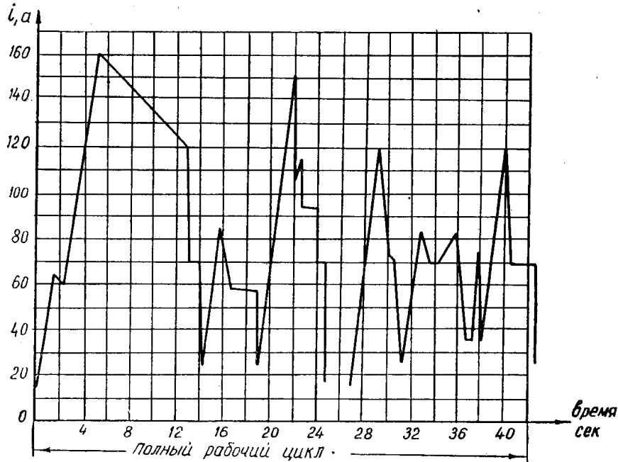
Рис. 2. График тока нагрузки экскаватора за рабочий цикл
