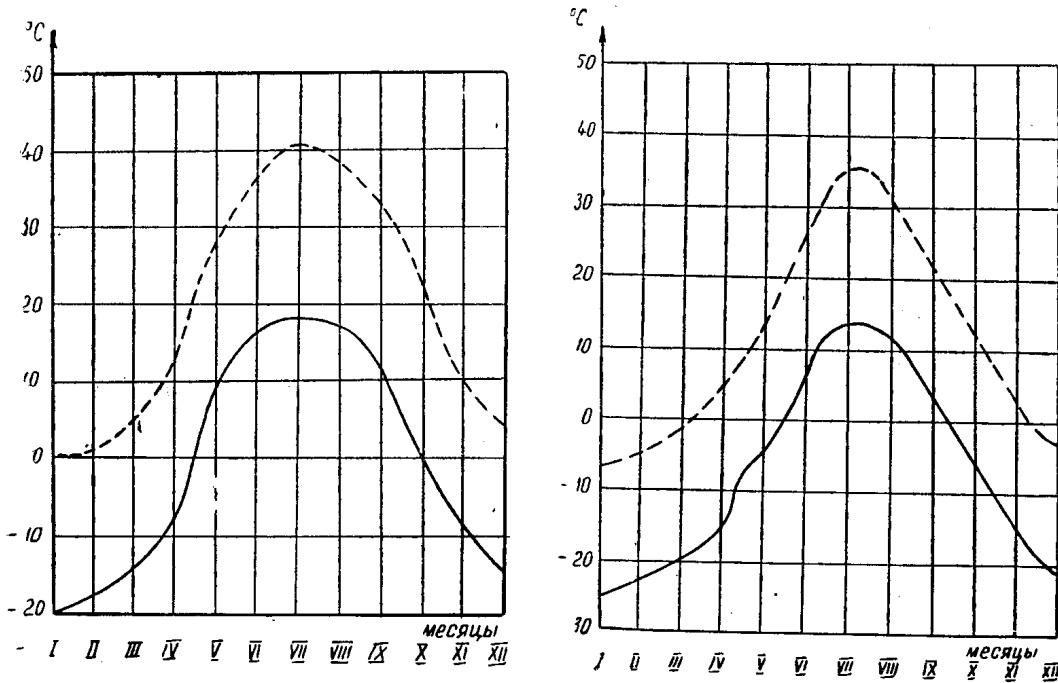
Рис. 3. Годовой график температур: _____ окружающей среды; - - - - - изоляции кабеля при сечении токопроводящей жилы 25 мм 2
