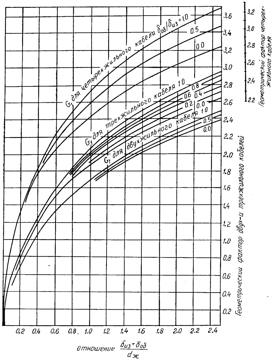
Рис. 1. Геометрический фактор G_1 для кабелей: \delta_{из} — толщина изоляции, \delta_{об} — толщина оболочки, d_{ж} диаметр токопроводящей жилы
