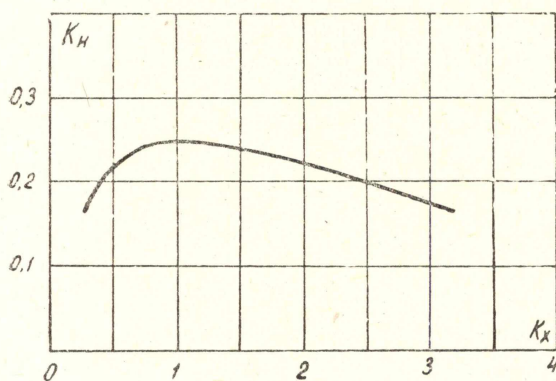
Рис. 1. Зависимость k_n в функции от k_x
