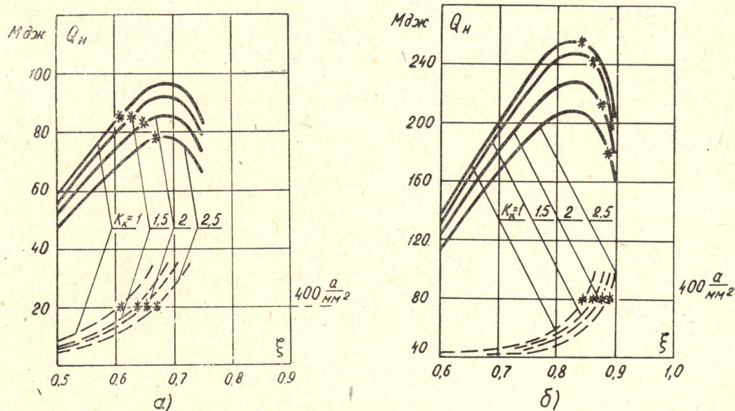
Рис. 2. Зависимость энергии и плотности тока в функции при k_1=2 и q=6 : а) для 8-полюсной машины с f=50 гц; б) для 2-полюсной машины с f=12,5 гц
