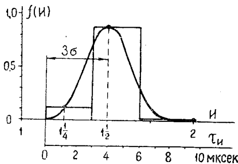
Рис. 1. Гистограмма распределения уровней искрения машин серии П 1-6 габаритов
