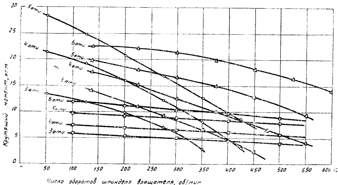
Рис. 2. Крутящий момент вращателей длинноходовых пневматических сверл типа СПВ: □ — с ротационным, ○ — с поршневым, △ — с шестеренчатым двигателем вращения бура.
