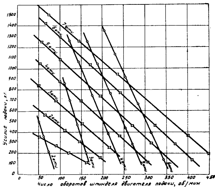
Рис. 3. Зависимость между усилием и скоростью подачи податчиков: ○—однозаходный винтовой механизм подачи сверла СПВ-1Д, □—четырезаходный винтовой механизм подачи сверла СПВ-2Д.
