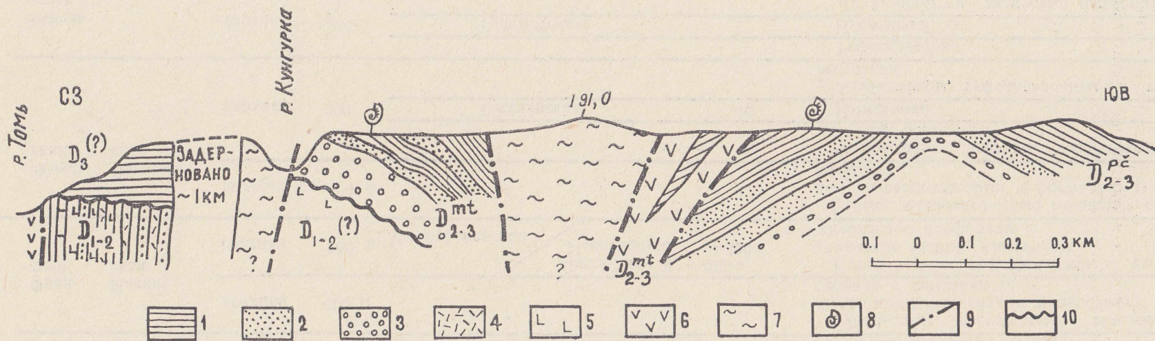
Рис. 1. Геологический разрез у ЮЗ окраины д. Митрофаново (правый берег р. Томи). 1 — сланцы; 2 — песчаники, алев-ролиты, 3 — конгломераты; 4 — туфы; 5 — альбитофиры; 6 — диабазы; 7 — кварциты; 8 — местонахождение фауны; 9 — разломы; 10 — размыв.
