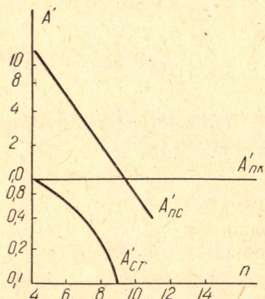
Рис. 1. Относительные информационно-аппаратурные критерии АЦП
