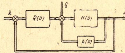
Рис. 1. Матричная структурная схема СМР
