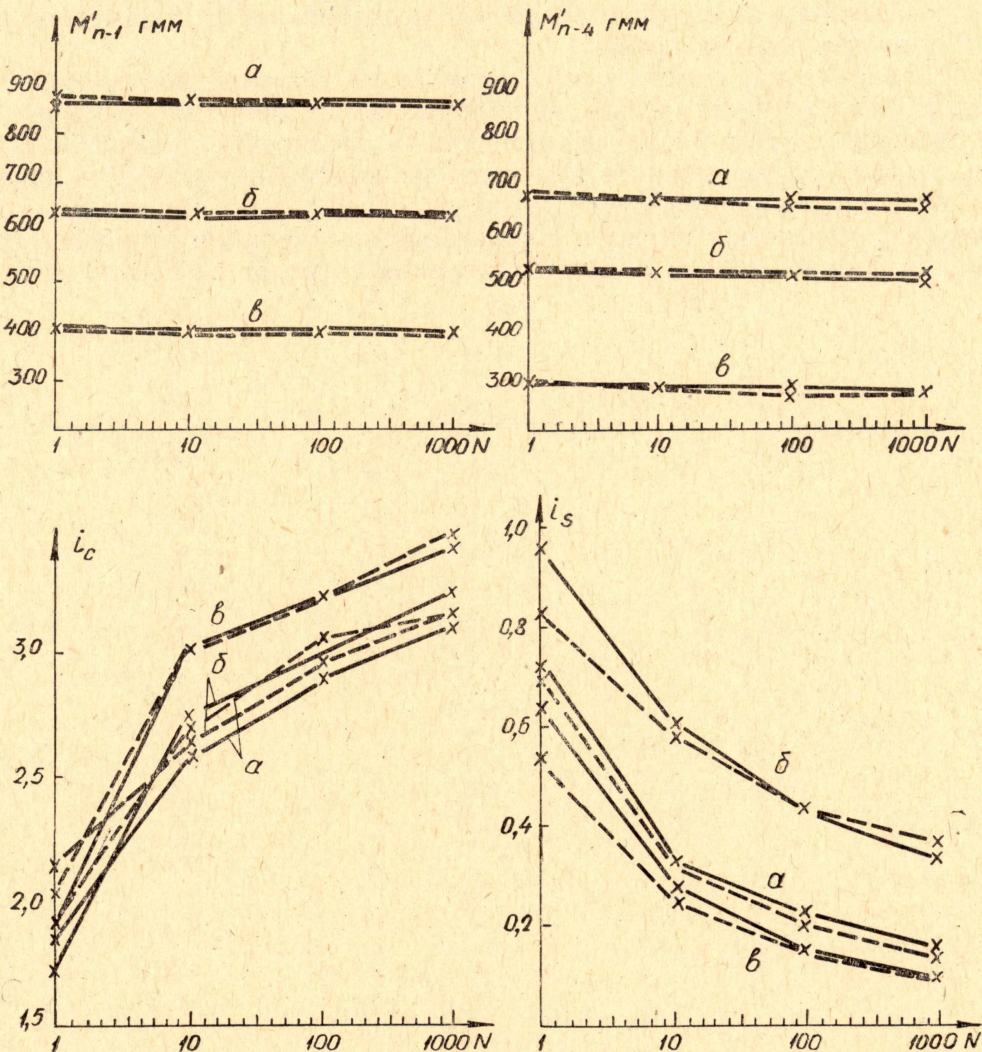
Рис. 2. Крутящие моменты M'_{n-1} , M'_{n-4} , прямые i_c и обратные i_s витки в зависимости от числа циклов завод-спуск при различной продолжительности второго заневольивания в сутках: ————— 0 суток, ———— 10 суток; а-пружины 0,085 \times 1,35 \times 220 мм; б-пружины 0,105 \times 1,38 \times 325 мм; в-пружины 0,12 \times 1,50 \times 335 мм
