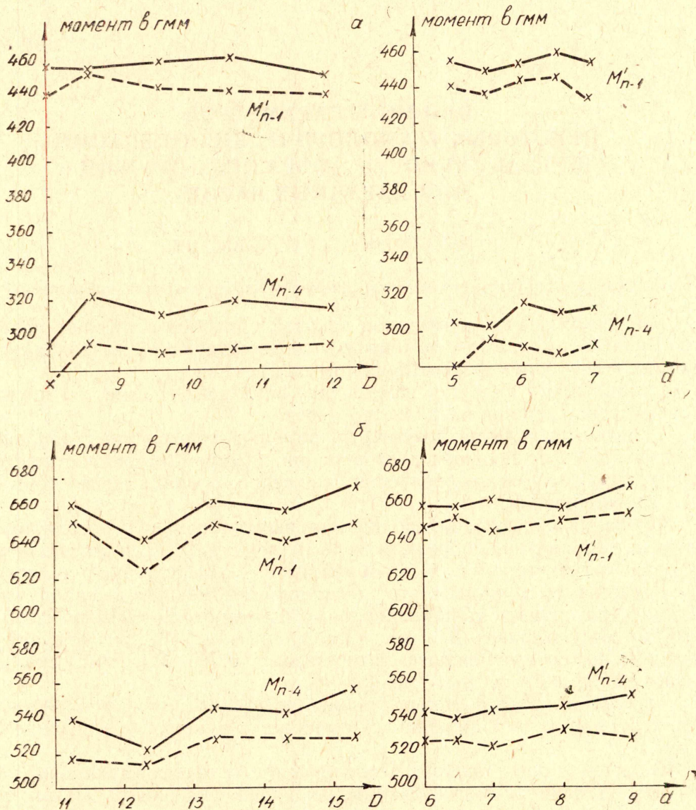
Рис. 1. Крутящие моменты M'_{n-1} , M'_{n-4} пружин в зависимости от диаметра D кольца для первого заневольивания и диаметра d валика для обратной навивки: а-пружины 0,085 \times 1,35 \times 220 мм; б-пружины 0,105 \times 1,38 \times 325 мм; _____ N=0 , - - - - - N=1000 циклов завод-спуск
