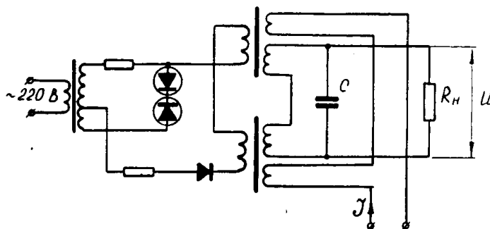
Рис. 1. Схема для экспериментального исследования параметрического усилителя.
