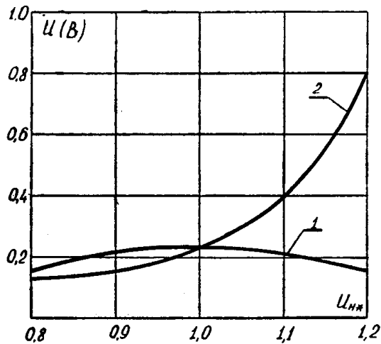
Рис. 3. Зависимости напряжения на контуре параметрического усилителя: 1 — при наличии стабилизации; 2 — без стабилизации.
