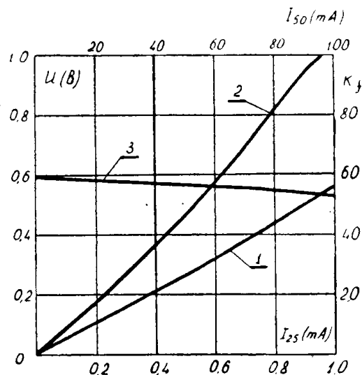
Рис. 2. Зависимости напряжения на контуре параметрического усилителя от тока в сигнальной обмотке: 1 — с частотой 25 Гц; 2 — с частотой 50 Гц; 3 — коэффициент отстройки по частоте.
