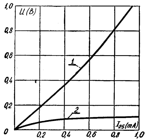
Рис. 4. Напряжение на контуре при фазах накачки, соответствующих максимальному (1) и минимальному усилению (2).
