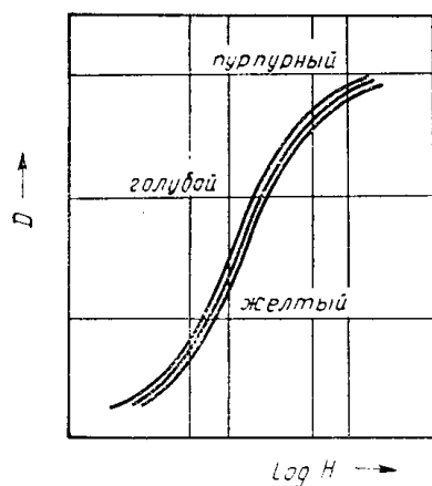
Рис. 3. Характеристические кривые цветного материала, сбалансированного по светочувствительности и контрасту. D — цветовая оптическая плотность; H — интенсивность освещения.
