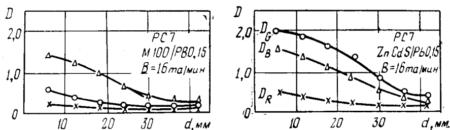
Рис. 5. Частичные плотности цвета пленки ORWO color PC7 при различных комбинациях экранов при просвечивании Al. D_B — цветовая плотность за синим фильтром; D_G — цветовая плотность за зеленым фильтром; D_R — цветовая плотность за красным фильтром.
