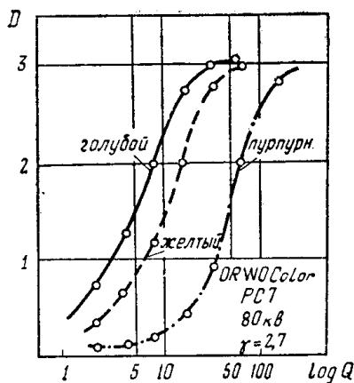
Рис. 4. Характеристические кривые позитивной пленки ORWOcolor PC7 при просвечивании ее x-лучами ( U=80 кВ). D — цветовая оптическая плотность; Q — интенсивность x-лучей.
