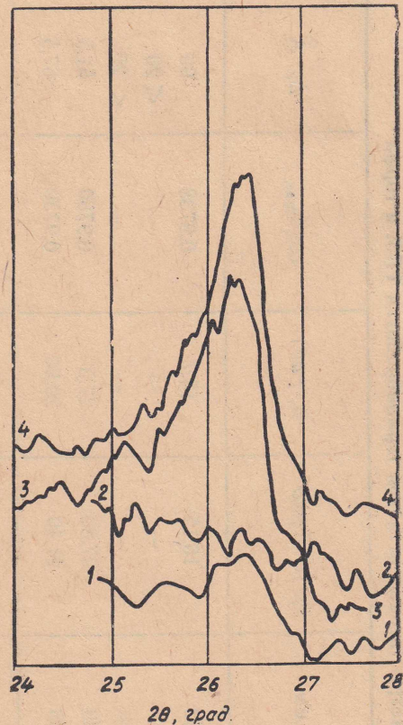
Рис. 2. Рентгенограммы ТФМ. 1 — исходный, М-1:1; 2 — 800^\circ\text{C} , М-1:2; 3 — 1000^\circ\text{C} , М-1:2; 4 — 1200^\circ\text{C} , М-1:2
