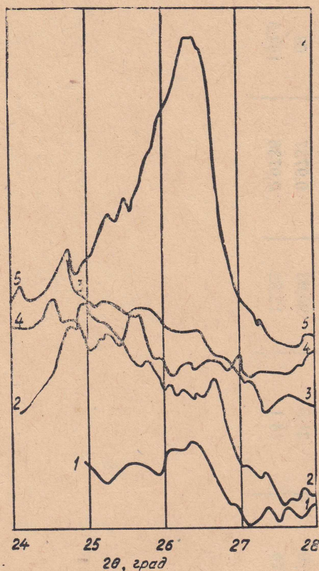
Рис. 1. Рентгенограммы торфа. 1 — исходный торф, М-1:1; 2 — 400^\circ\text{C} , М-1:1; 3 — 800^\circ\text{C} , М-1:1; 4 — 1000^\circ\text{C} , М-1:2; 5 — 1200^\circ\text{C} , М-1:2
