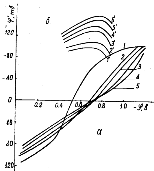
Рис. 1. Кривые \Psi' — \Phi , рассчитанные: а) по формуле (1), б) по формуле (2). Содержание \beta -нафтола в растворе моль/л \times 10^4 : 1) 0,00; 2) 1,22; 3) 2,44; 4) 6,1; 5) 12,2; 1) 1,83; 2) 2,44; 3) 4,88; 4) 7,32; 5) 9,76; 6) 12,2
