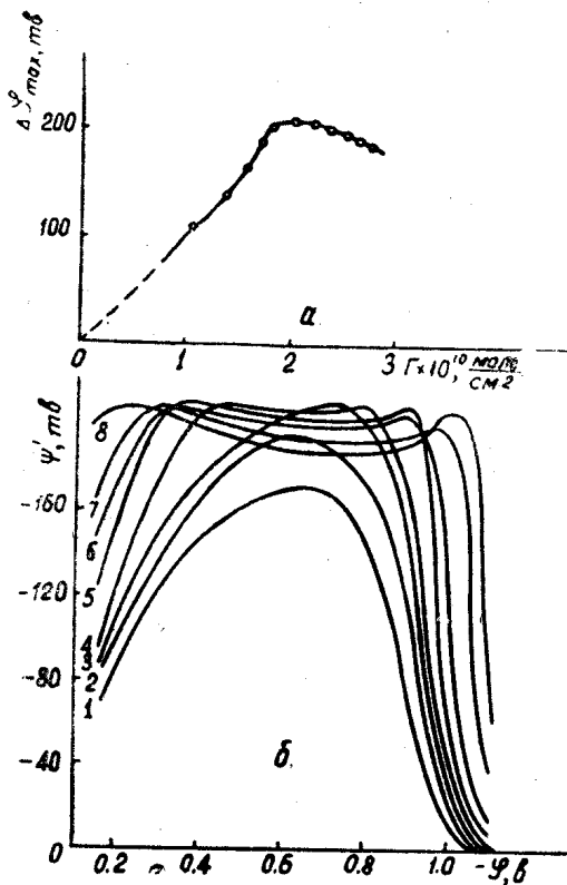
Рис. 2. Зависимость сдвига максимума электрокапиллярной кривой от количества адсорбированного вещества (а) и рассчитанные по ней \Psi' , \Phi — кривые (б) для концентраций \beta -нафтола, моль/л \times 10^4 : 1) 1,22; 2) 1,83; 3) 2,44; 4) 3,66; 5) 6,1; 6) 7,32; 7) 9,76; 8) 12,2
