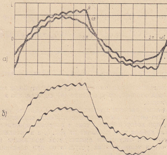
Рис. 5. Кривые тока в нагрузке при k=10 и \cos\varphi=0,8 : а — расчетные кривые, б — экспериментальные осциллограммы
