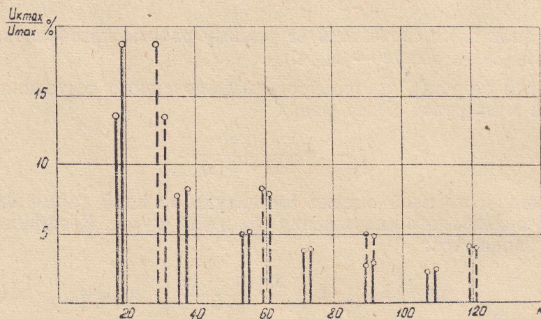
Рис. 3. Зависимость амплитуд высших гармонических от номера гармоник для \nu=4 и m=6 при f_{\text{пер}} < f_{\text{вх}} (сплошная линия) и f_{\text{пер}} > f_{\text{вх}} (штриховая линия)
