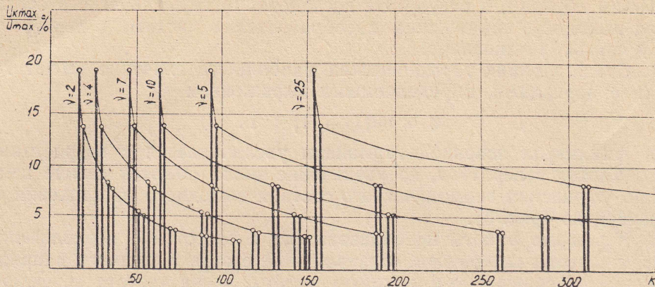
Рис. 4. Спектральный состав выходного напряжения преобразователя частоты для f_{пер} > f_{вх} при различных \nu
