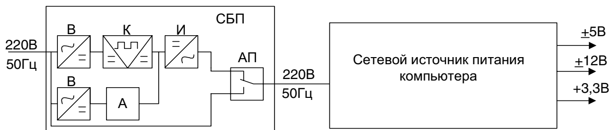
Рис. 2. Структура СБП типа on-line
