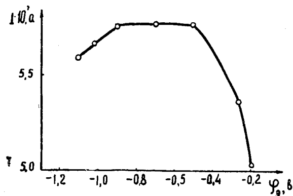
Рис. 2. Зависимость тока электрорастворения иридия (+4) от потенциала накопления
