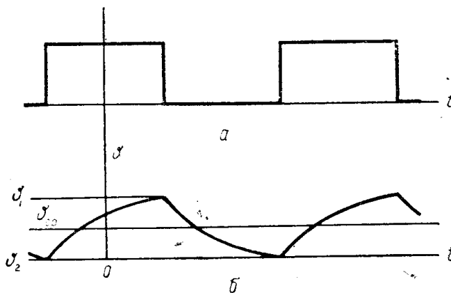
Рис. 1. a — тепловое воздействие, b — температура, \vartheta — \vartheta — зона нечувствительности регулятора.
