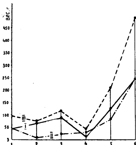
Рис. 1. Количество вещества, перемещенного при формировании зон метасоматической колонки в контактах даек габбро (в граммах на 100 \text{ см}^3 породы). I — привнос, II — вынос, III — суммарное количество перемещенного вещества: 1. Замещение габбро скаполитовой породой. 2. Замещение скаполитового метасоматита гранатовым. 3. Замещение волластонитового метасоматита гранатовым. 4. Замещение волластонит-альбит диопсидового метасоматита волластонитовым. 5. Замещение кварцевого метасоматита волластонит-альбит-диопсидовым. 6. Замещение известняка кварцевым метасоматитом.
