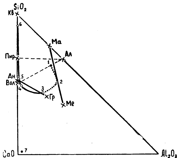
Рис. 2. Диаграмма состав-парагенезис для метасоматических образований в контактах даек габбро: 1. Габбро. 2. Скаполитовая порода. 3. Гранатевая порода. 4. Волластонитовая порода. 5. Волластонит - альбит - диопсидовая порода. 6. Кварцевая порода. 7. Известняк вмещающей толщи. Ал-альбит. Ан-андрадит. Гр-гроссуляр. Вол-волластонит. Кв-кварц. Пир-диопсид. Ма-марриалит. Мс-мейонит. Точками соединены химические составы эндоконтактовых образований, сплошной линией — составы экзоконтактовых образований.
