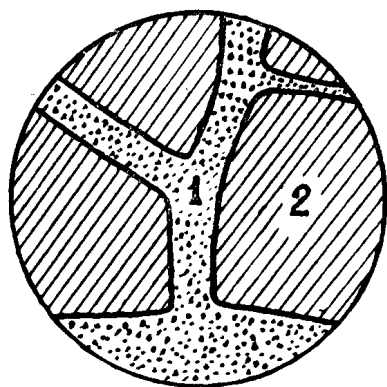
Рис. 1. Метасоматические жилки серпентина и диопсида (1) в биотитизированном трахидолерите (2).
