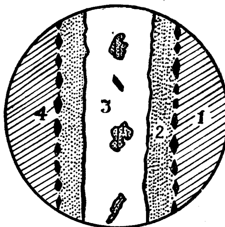
Рис. 2. Строение метасоматических жилок: биотитизированный трахидолерит (1); зона диопсида с псевдоморфозами серпентина по плагиоклазу (2); полоса серпентина с крупными зернами диопсида и сфена (3); цепочка зерен сфена (4).
