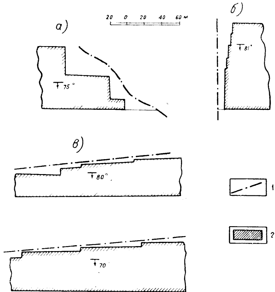
Рис. 1. Отработка угольных пластов у тектонических разрывов (а — диагональных, б — поперечных, в — продольных) 1) обрез пласта тектоническим разрывом; 2) отработанные участки пласта.
