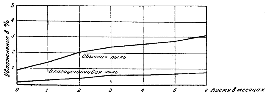
Рис. 2. Увлажнение пыли на полке заслона в зависимости от времени
