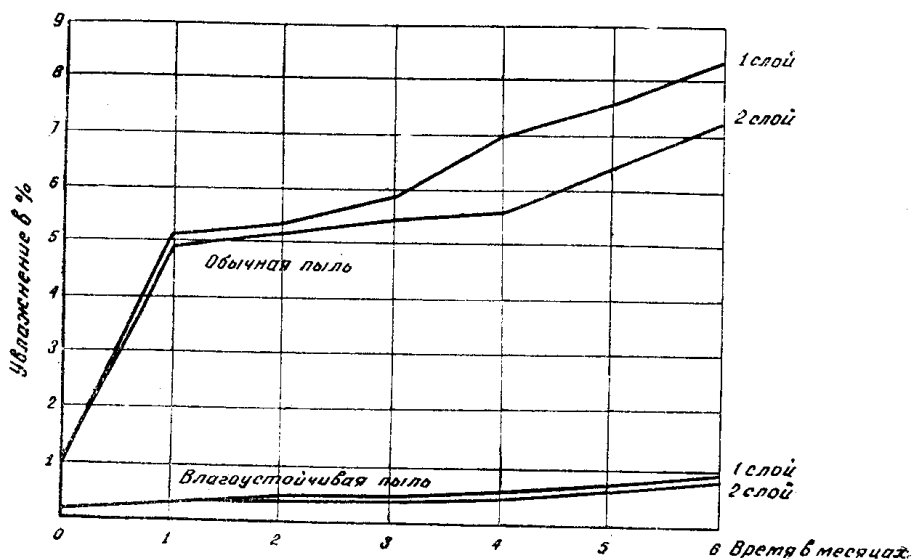
Рис. 3. Увлажнение пыли в слоях в зависимости от времени
