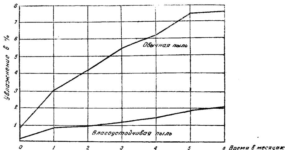
Рис. 1. Динамика увлажнения пыли в зависимости от времени
