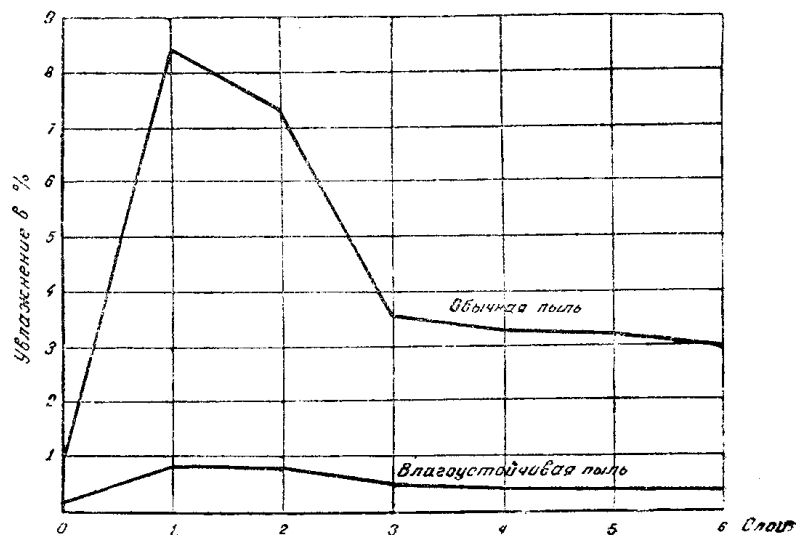
Рис. 4. Увлажнение пыли по слоям через 6 месяцев
