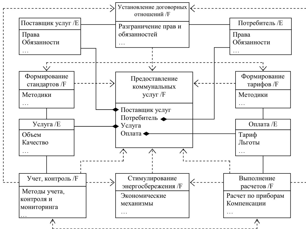
Рис. 1. Объектная модель системы предоставления коммунальных услуг
