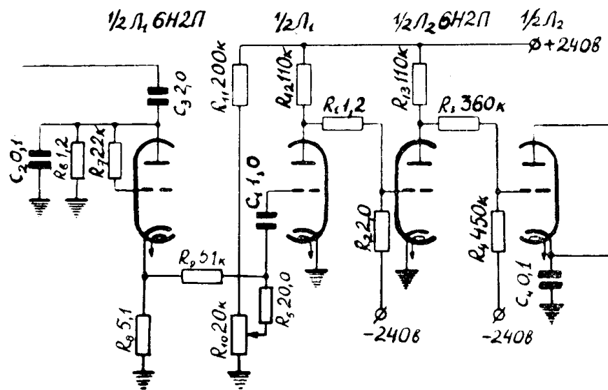
Рис. 1. Схема приставки к осциллографическому полярографу ОП-1 или ОП-2.
