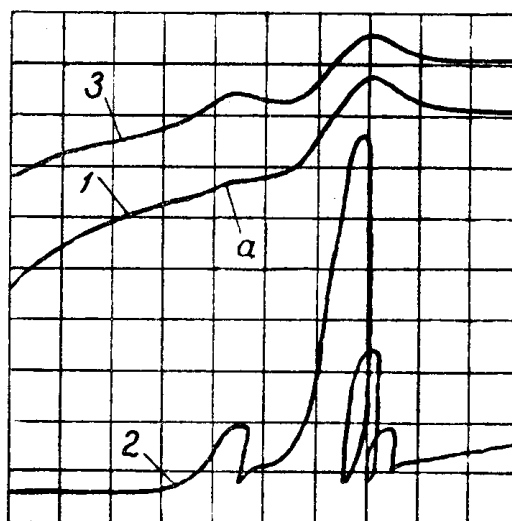
Рис. 2. Пики кадмия и таллия при совместном присутствии (условия см. табл. 1): 1, 3 — без приставки; 2 — с приставкой.
