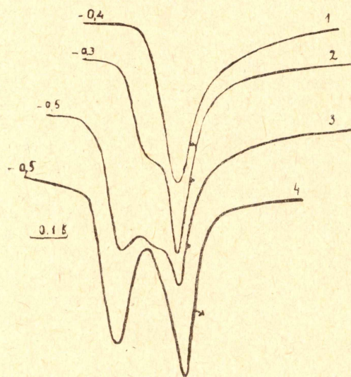
Рис. 3. Типичные формы простого и сложных зубцов меди на фонах: 1— 0,5 М K_2CO_3 ; 2— 0,1 М K_2CO_3 ; 3— 0,1 М KOH (электрод—капля ртути); 4— 0,1 М K_2CO_3 (пленочный электрод).
