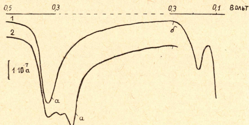
Рис. 5. Анодные полярограммы меди, снятые с остановкой потенциала после первого зубца (кривая 1) и второго зубца (2). Точками а и б обозначены моменты остановки и пуска потенциометрического барабана.
