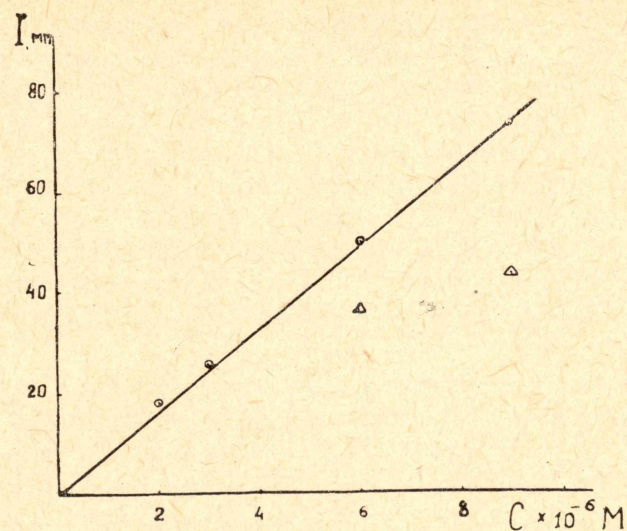
Рис. 1. Зависимость высоты второго зубца меди от концентрации ионов \text{Cu} (2+) в растворе 0,1 \text{ M K}_2\text{CO}_3 . Условия опыта: \tau = 3 \text{ мин} ; v = 5 \text{ мл} ; r = 0,04 \text{ см} ( \tau — время электролиза; v — объем раствора; r — радиус ртутной капли). Значком \triangle обозначена высота первого, более отрицательного зубца меди, появляющегося при концентрации \text{Cu} (2+) выше, чем 6 \cdot 10^{-6} \text{ M} .
