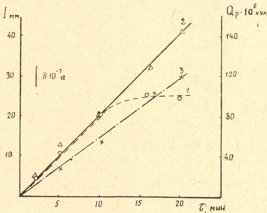
Рис. 2. Влияние времени предварительного электролиза на величину анодного тока первого (кривая 1) и второго (кривая 2) зубцов меди в 0,1 \text{ M KOH} . Кривая 3 — площадь под двойными зубцами меди с остановкой потенциала. Условия опыта: C = 1 \cdot 10^{-5} \text{ M} ; v = 5 \text{ мл} ; r = 0,04 \text{ см} ; W = 600 \text{ мв/мин} . ( C — концентрация меди в растворе).
